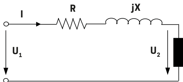
Circuito equivalente de una línea corta
